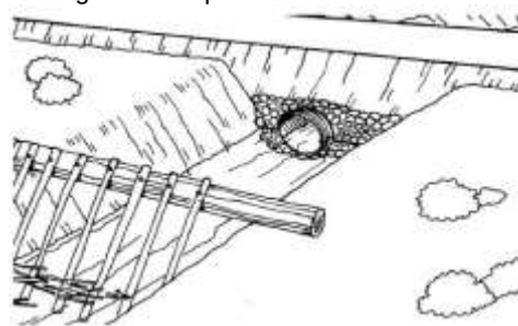
Figura 58: Ejemplo de rejilla para prevenir el ingreso de elementos grandes al paso de fauna acuática.
