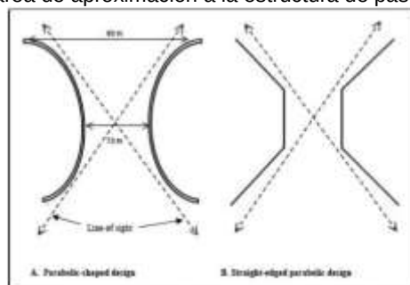
Figura 17: Opciones de diseño que aumentan el ancho del área de aproximación a la estructura de paso.
