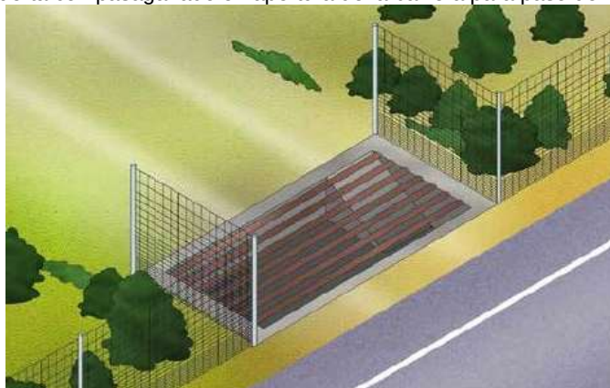
Figura 73: Puerta con pasaganado en apertura de la barrera para paso de fauna silvestre.
